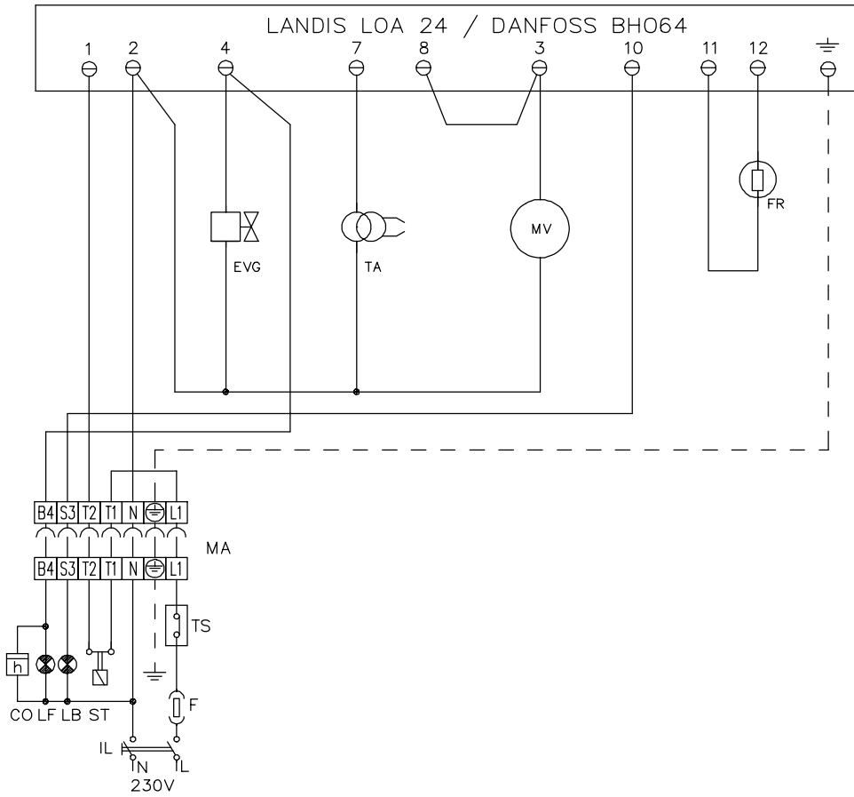
Esquema eléctrico (cód. 01-361) excluido G4 G-.TN.x.ES.A.P e G-.TN.x.ES.S
