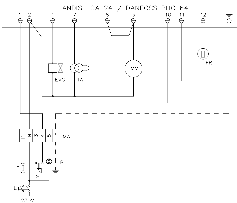
Esquema eléctrico (cód. 01-142/1) G4 G-.TN.x.ES.S
